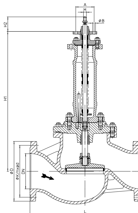
Fig. 460 DN200-250 M16
