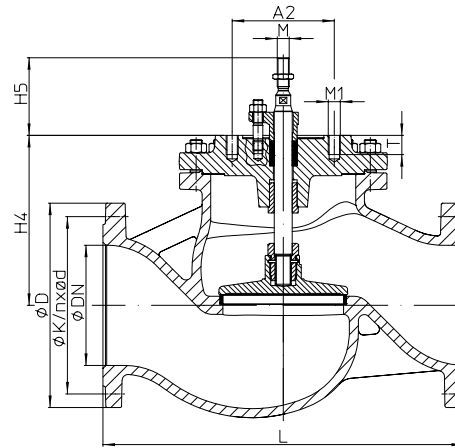
Fig. 405 DN125-250 M27 (e.g.: DP35; AUMA 14.2-14.6)
