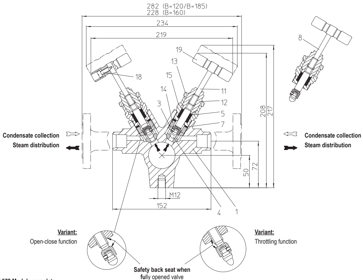
Fig. 671 / 672 Module complete
